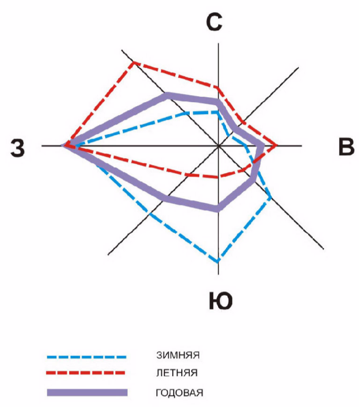
РОЗА ВЕТРА ПО НАПРАВЛЕНИЯМ В % ПО МЕТЕОСТАНЦИИ с.БАТЫРЕВО
