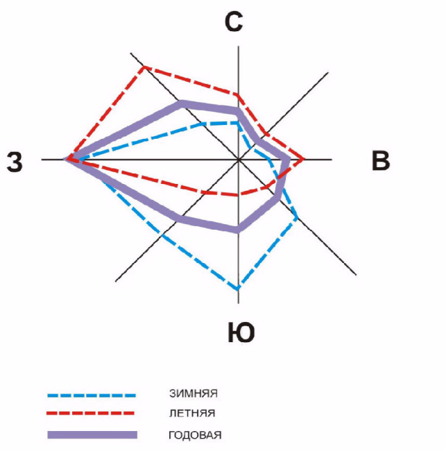
РОЗА ВЕТРА ПО НАПРАВЛЕНИЯМ В % ПО МЕТЕОСТАНЦИИ с.БАТЫРЕВО
