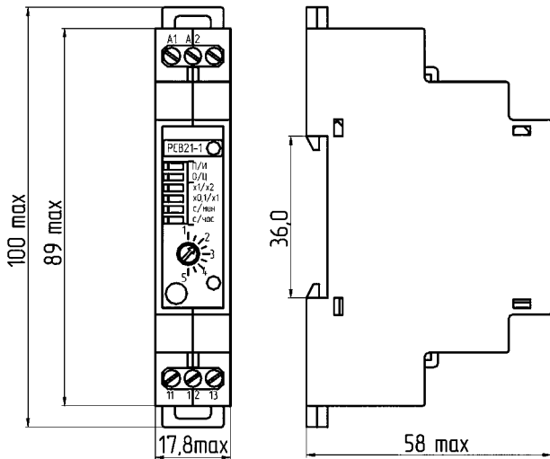
Рисунок 1. реле с креплением на DIN-рейку
