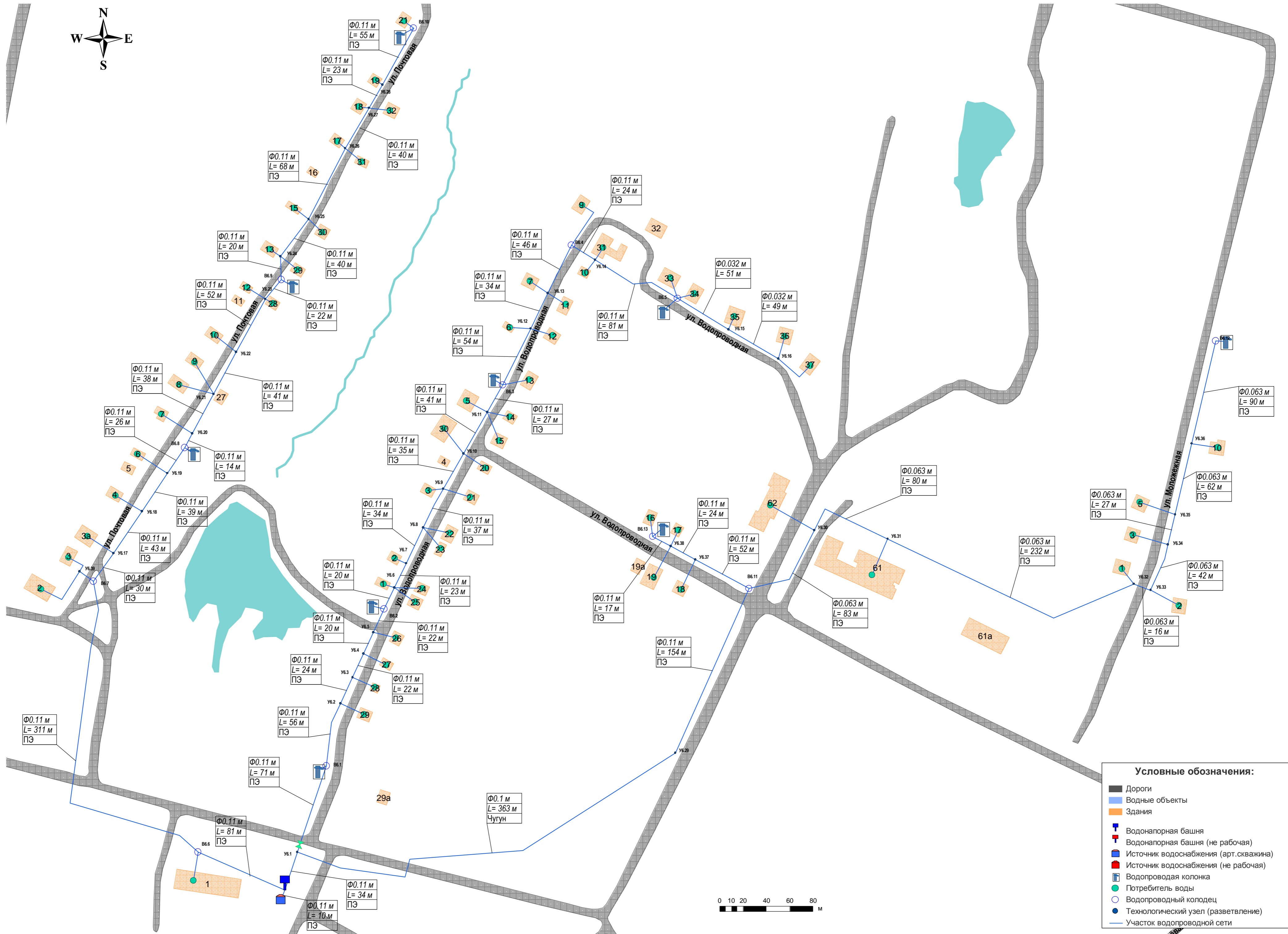
Приложение 1.5. Существующая схема водопроводной сети дер. Вурманкас-Туруново Чиршкасинского сельского поселения Чебоксарского района Чувашской Республики
