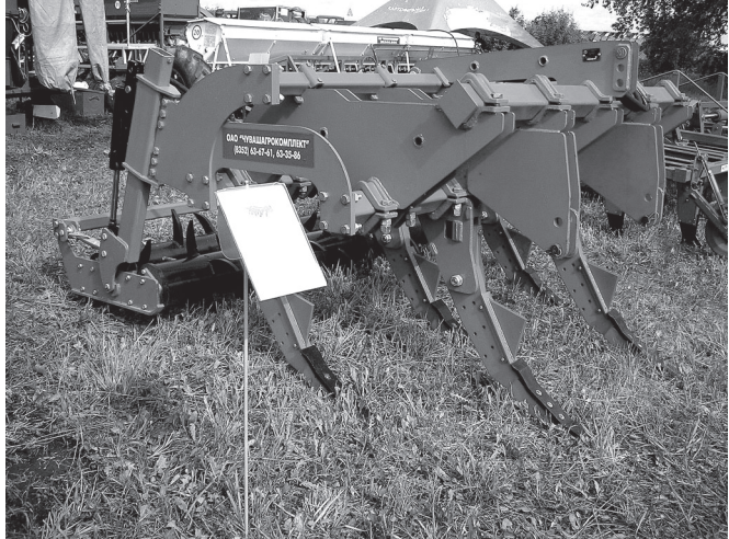
Сёре 65 см таранаш қалкалатан «Гаспардо ГН-2,5» сёр синче шыв тарасан пулашаты.
