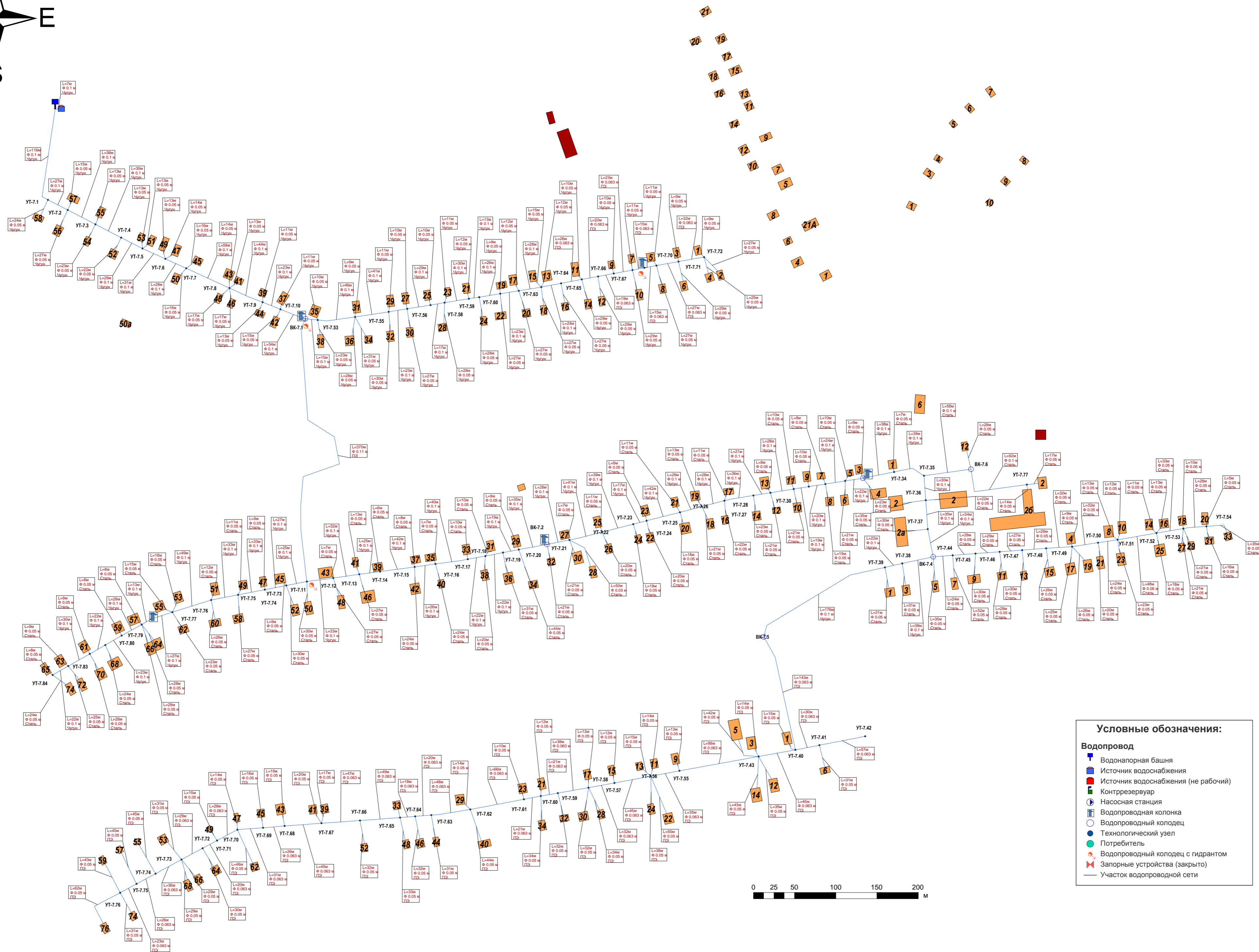
Приложение 1.4. Схема существующей водопроводной сети села Икково Сирмапосинского сельского поселения
