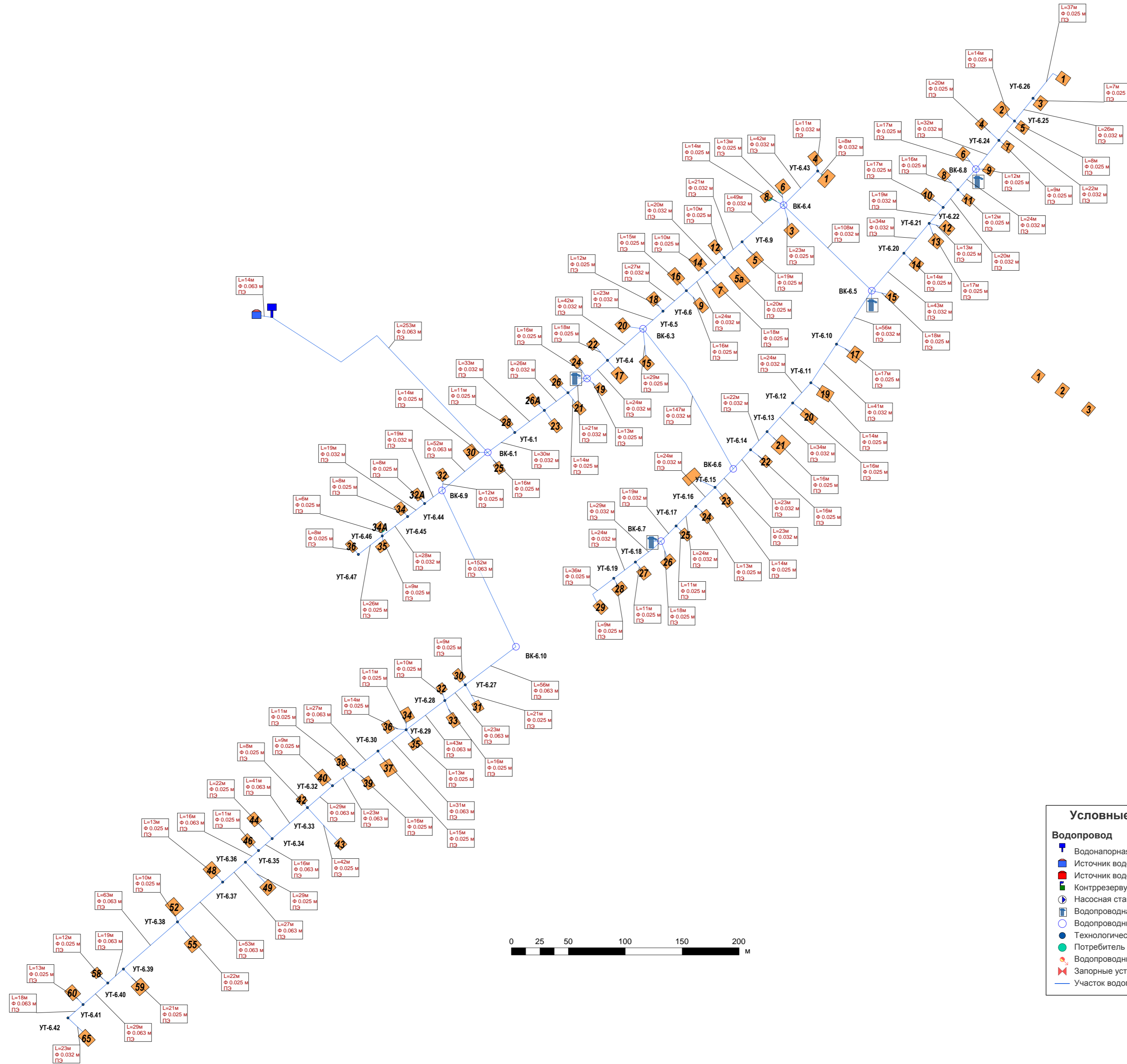
Приложение 1.3. Схема существующей водопроводной сети деревни Большое Янгильдино Сирмапосинского сельского поселения
